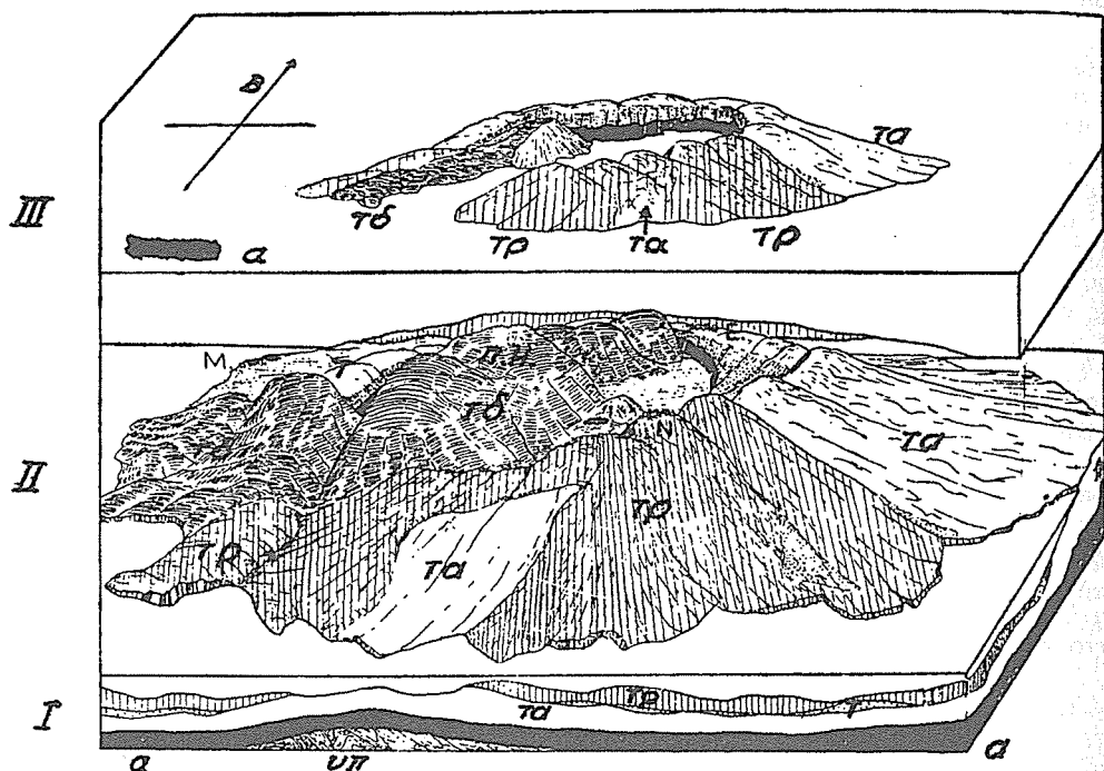
Σχ. 4.- Τὰ στάδια ἐξελίξεως τοῦ ἡφαιστείου τῆς Νισύρου (κατὰ τὸν Α. DESIO). Μ=Μανδράκι. Ε = Ἐμπορείος. Ν = Νικιά. Π.Η = Προφῆτης Ἡλίας. α = ἀνδесίται. τα = τραχυανδесίται. τρ = τραχεῖται. τδ=τραχειδακίται. Τὰ διὰ στιγμῶν σημειούμενα τμήματα εἶναι οἱ τόφφοι. ὑπ=τὸ ἐκ μὴ ἡφαιστειογενῶν πετρωμάτων ὑπόβαθρον τῆς νήσου.
