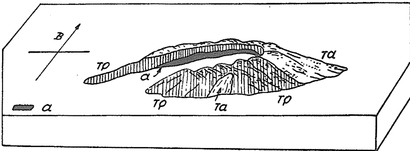
Σχ. 5— Τὰ πρώτα στάδια ἐξελιζέως τοῦ ἡφαιστείου. α = ἀνδεσίται. τα = τραχυανδεσίται, τρ = τραχεΐται.
