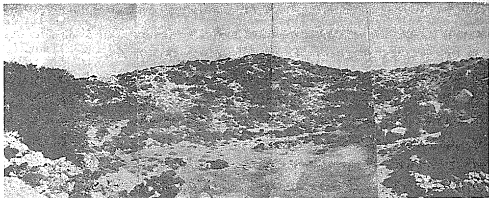
Σχ. 8.— Τὸ ἐγκατακρημνισιγενὲς κρατηροειδὲς κοίλωμα ἐπὶ τῆς κορυφῆς τοῦ ἡφαιστείου θόλου τοῦ Προφ. Ἡλίου (Διαβάτη).
