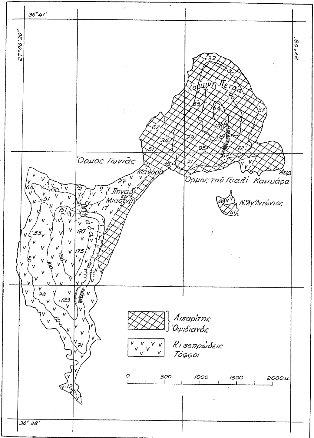
Σχ. 2.— Γεωλογικός χάρτης της νησίδος Γαλι (κατά τὸν Α. Μαρτελλί).
